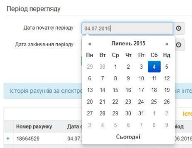
Рисунок 7. Вибір дати
